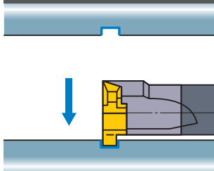
1 Угловой тип (FSL5208R,5210R)
