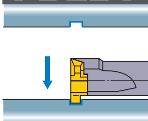
1 Угловой тип (FSL5108R,5110R)
